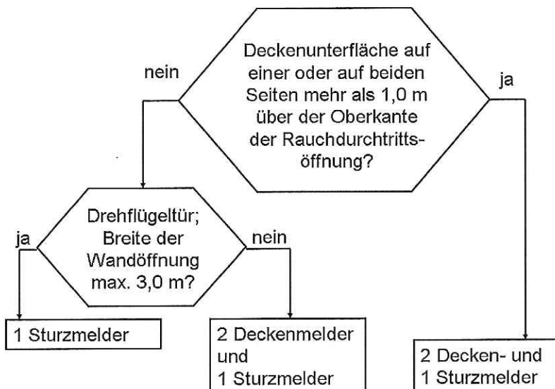
Bild 3: Entscheidungsdiagramm
